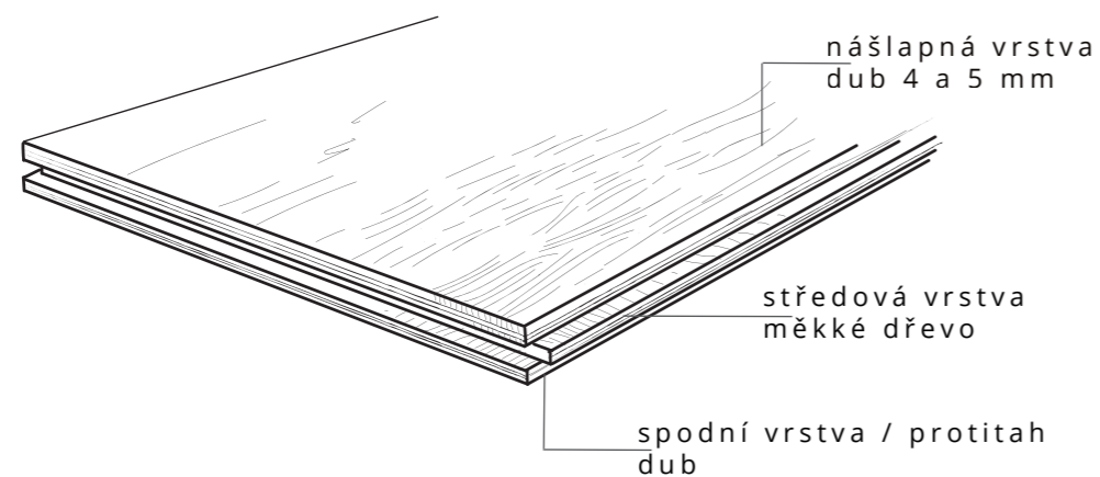
SPOJ PERO-DRÁŽKA
